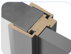
Короб телескоп, наличник Тип 1
