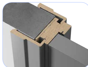
Короб телескоп, наличник Тип 2
