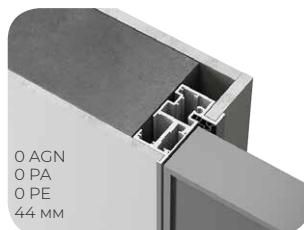
Короб INVISIBLE / INFINITY
