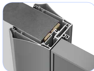
Короб INTEGRAL, наличник Фигурный
